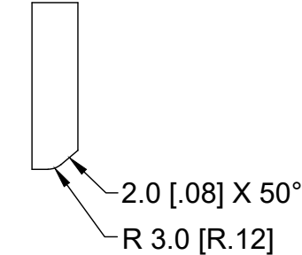
DETAIL C SCALE 1:1 OPTIONAL EDGE
